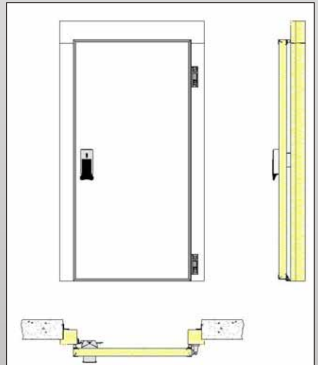
Yükselen Menteşe Sistemi Cam Hinge System
