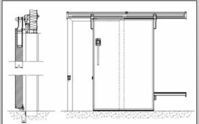
Eksenel Kuyruk Sistemi Axis Rear System
